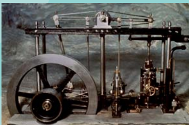
Maszyna parowa Jamesa Watta
